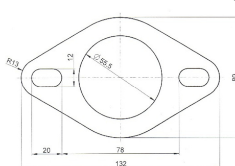
FLANSZA/ FLANGE/FLANSCH/ ФЛАНЕЦ
