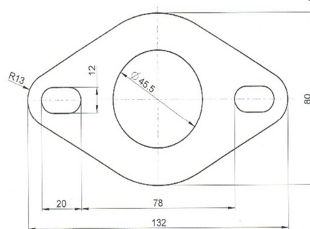
FLANSZA/ FLANGE/FLANSCH/ ФЛАНЕЦ
